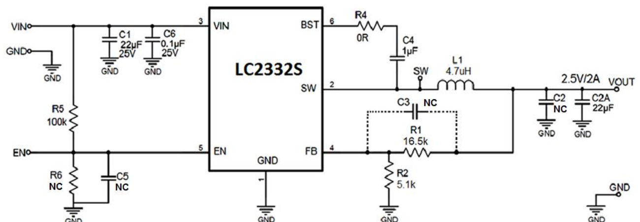
Figure3. 12V VIN, 2.5V/2A
