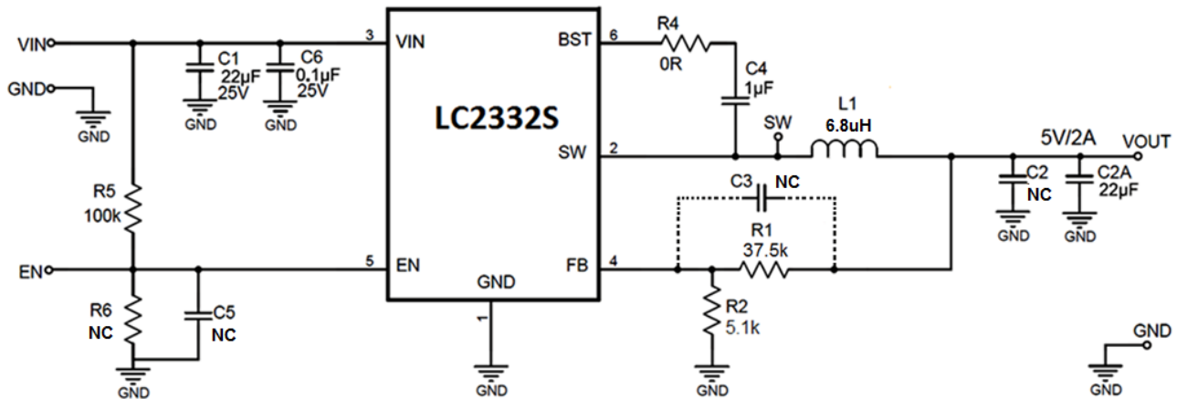
Figure1. 12V VIN, 5V/2A
