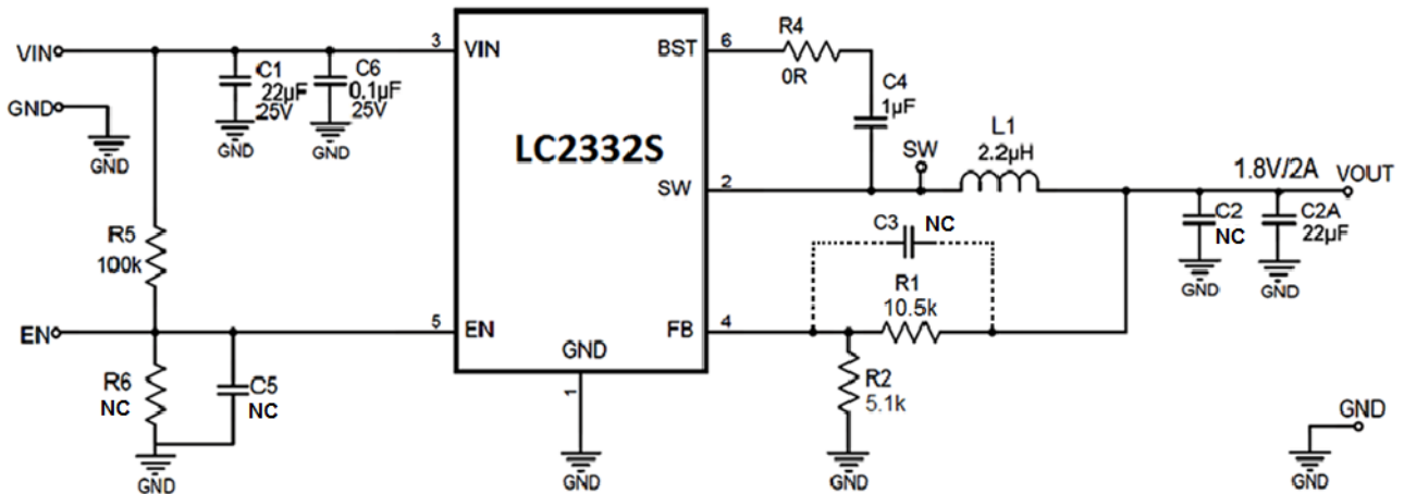
Figure4. 12V VIN, 1.8V/2A
