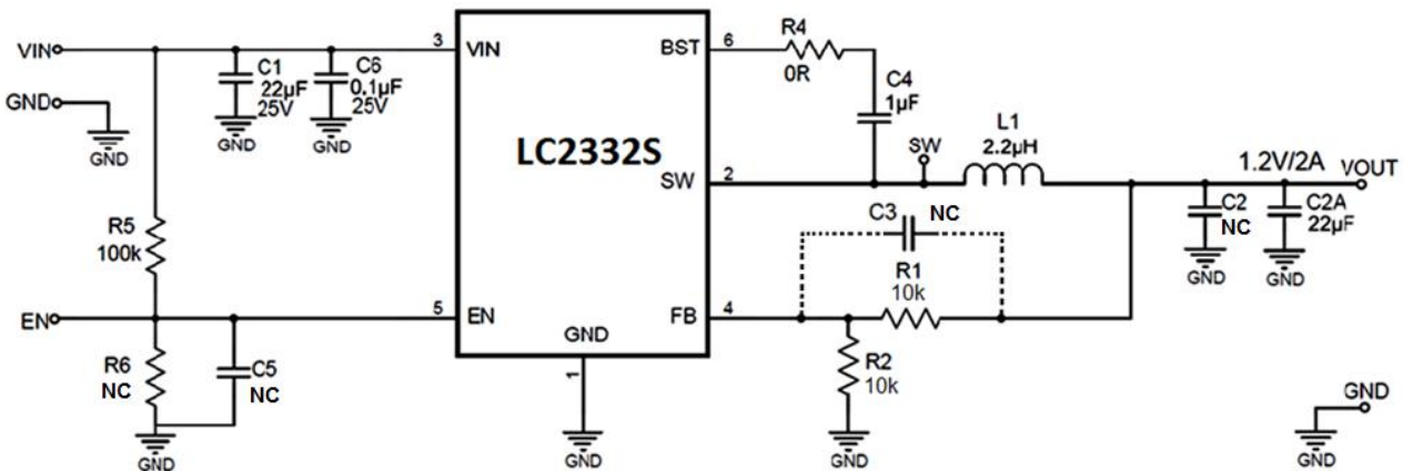
Figure5. 12V VIN, 1.2V/2A
