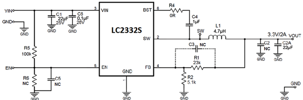
Figure2. 12V VIN, 3.3V/2A
